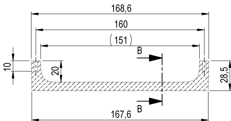
ŘEZ A-A
