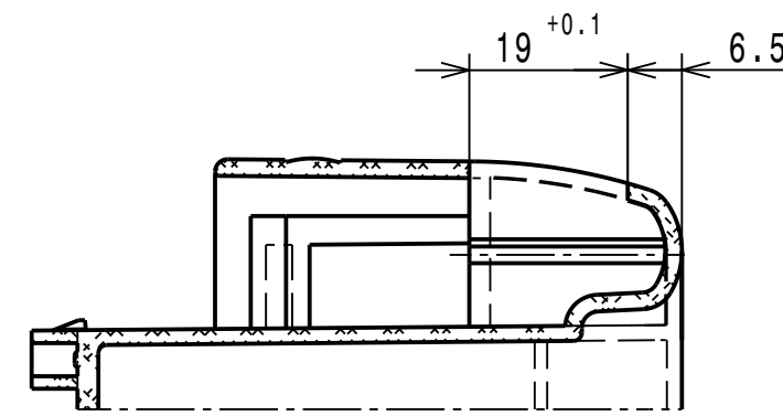
Schnitt F-F
