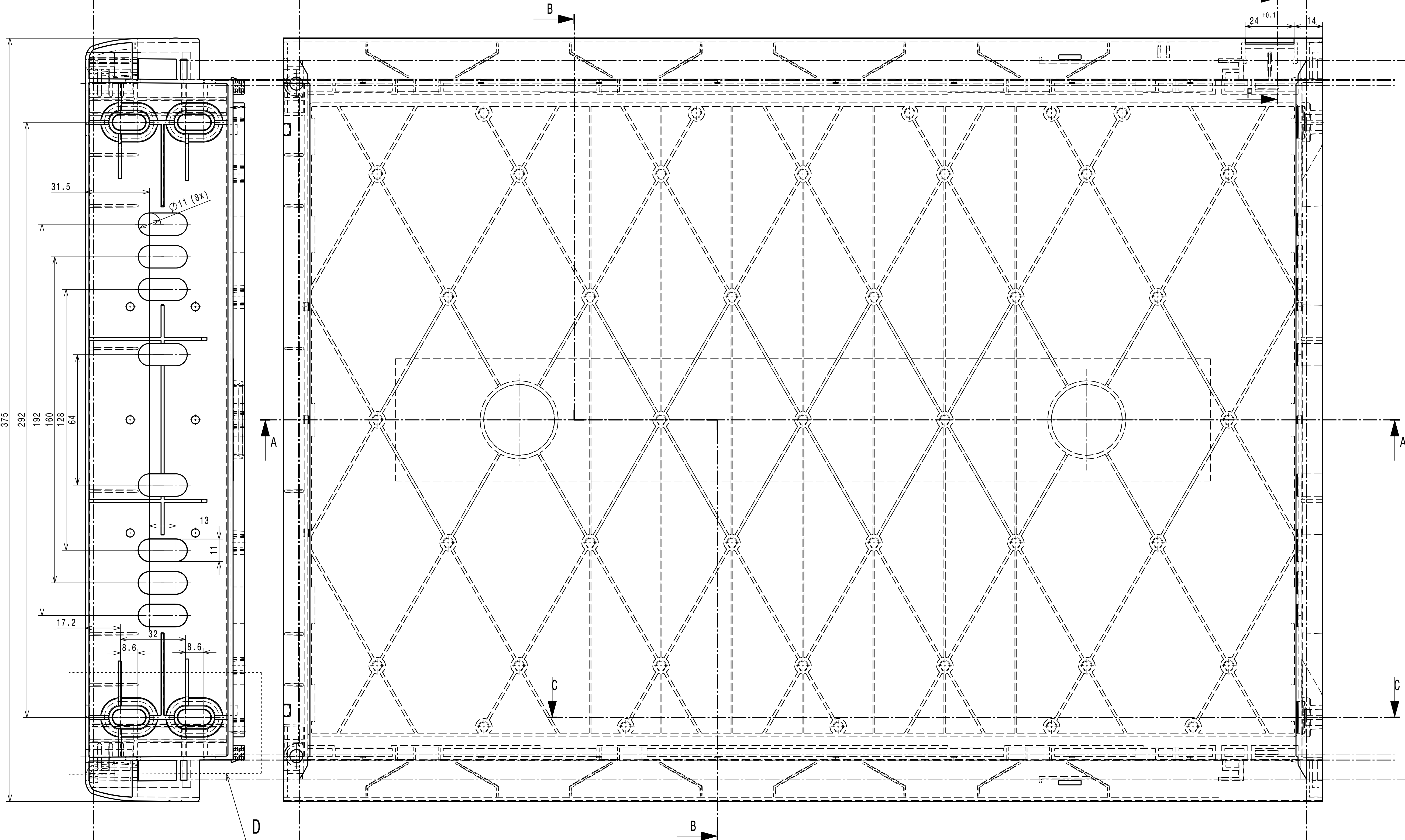
Detail D M 2:1
