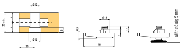
szerelés a Target J12 rendszerrel kombinálva
