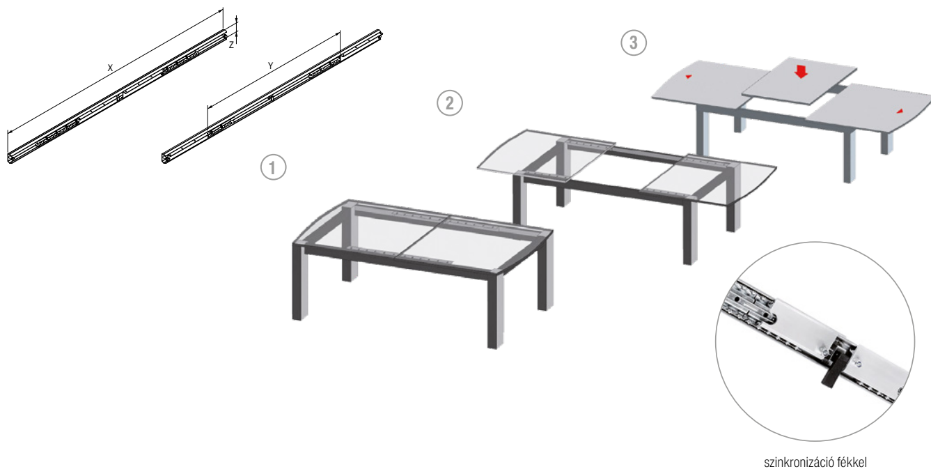
szinkronizáció fékkel
