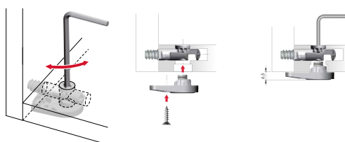
szerelés a Target J12 rendszerrel kombinálva
