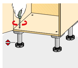
Magasság beállítása fentről csavarhúzóval.
