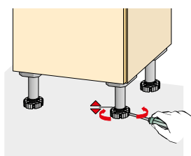
Magasság beállítása az előlő oldalról csavarhúzóval.
