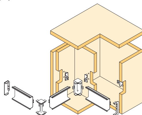
Vízszintes fiók „C” profil.
